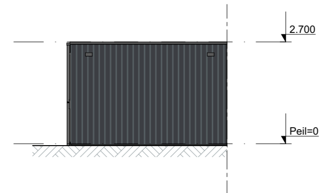
Buitenberging - Type 1 Dubbel GVL - Linkergevel
