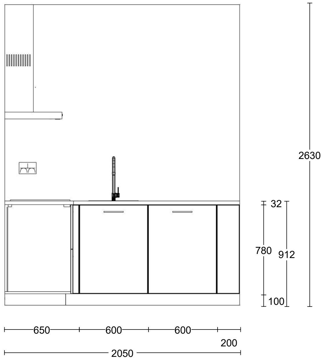
Vooraanzicht wand 2
