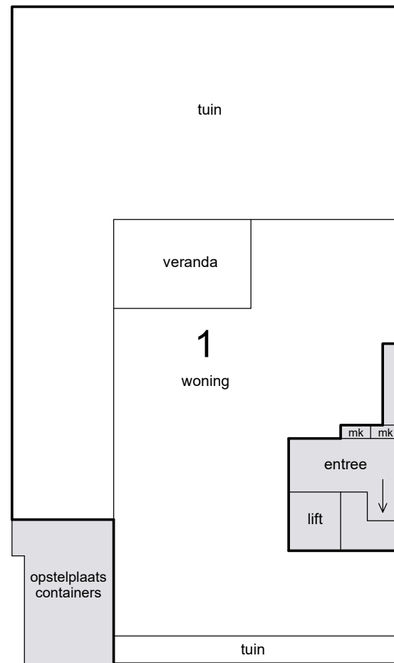
begane grond
