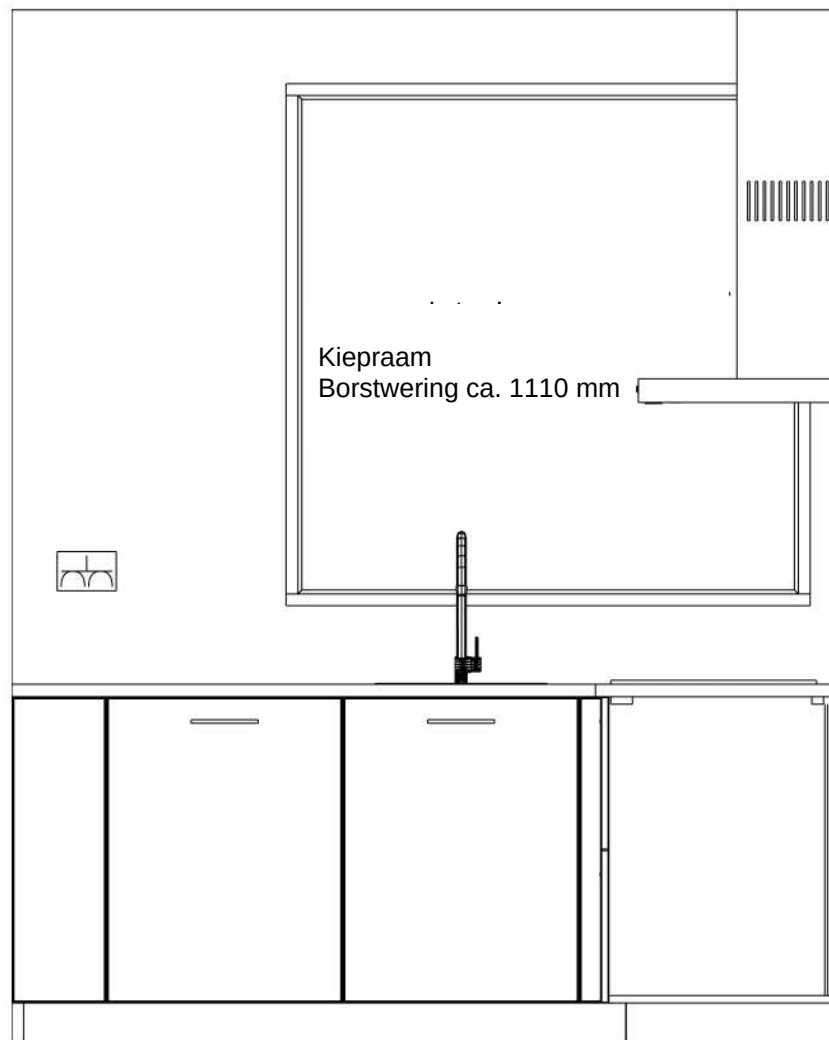
Vooraanzicht wand 1
