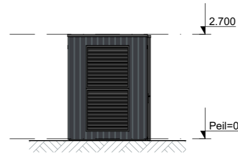
Buitenberging - Type 3 Dubbel GVL - Voorgevel
