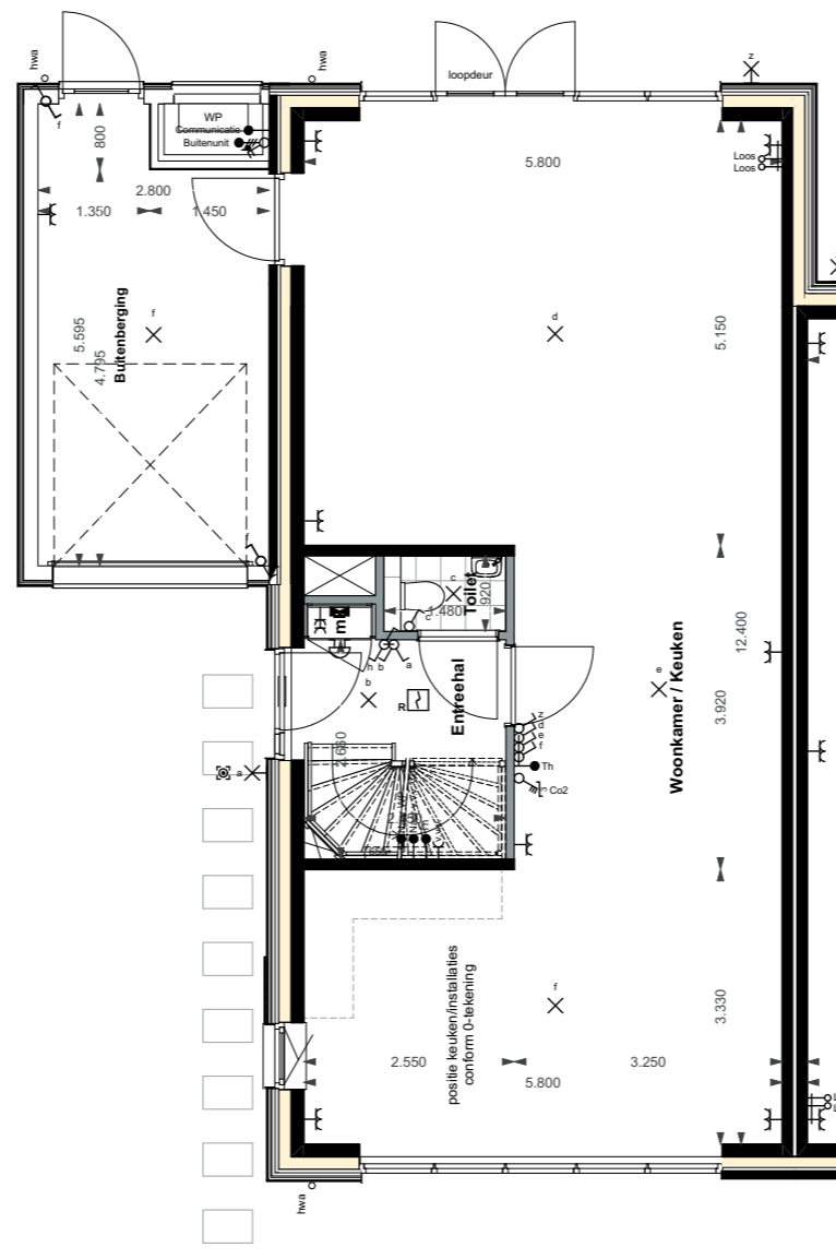
1.A.0.34 | Uitbouw achtergevel 240 cm
