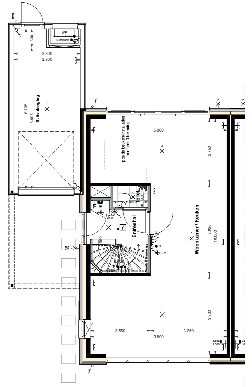
1.A.0.36 | Verlengen ongeïsoleerde berging 120 cm
