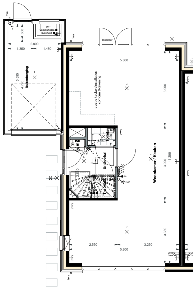
1.A.0.32 | Uitbouw achtergevel 120 cm
