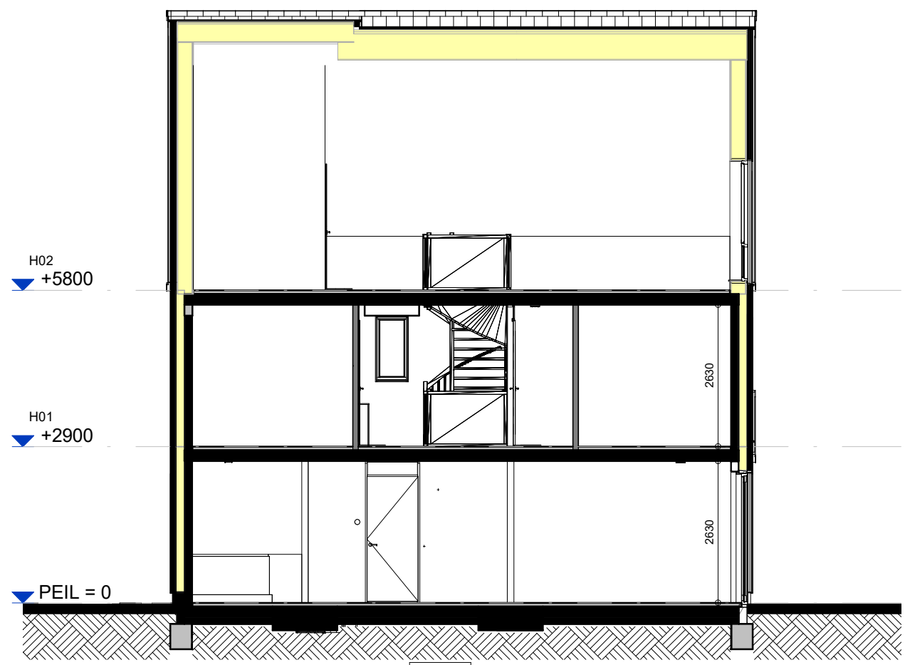
Doorsnede V02 145
