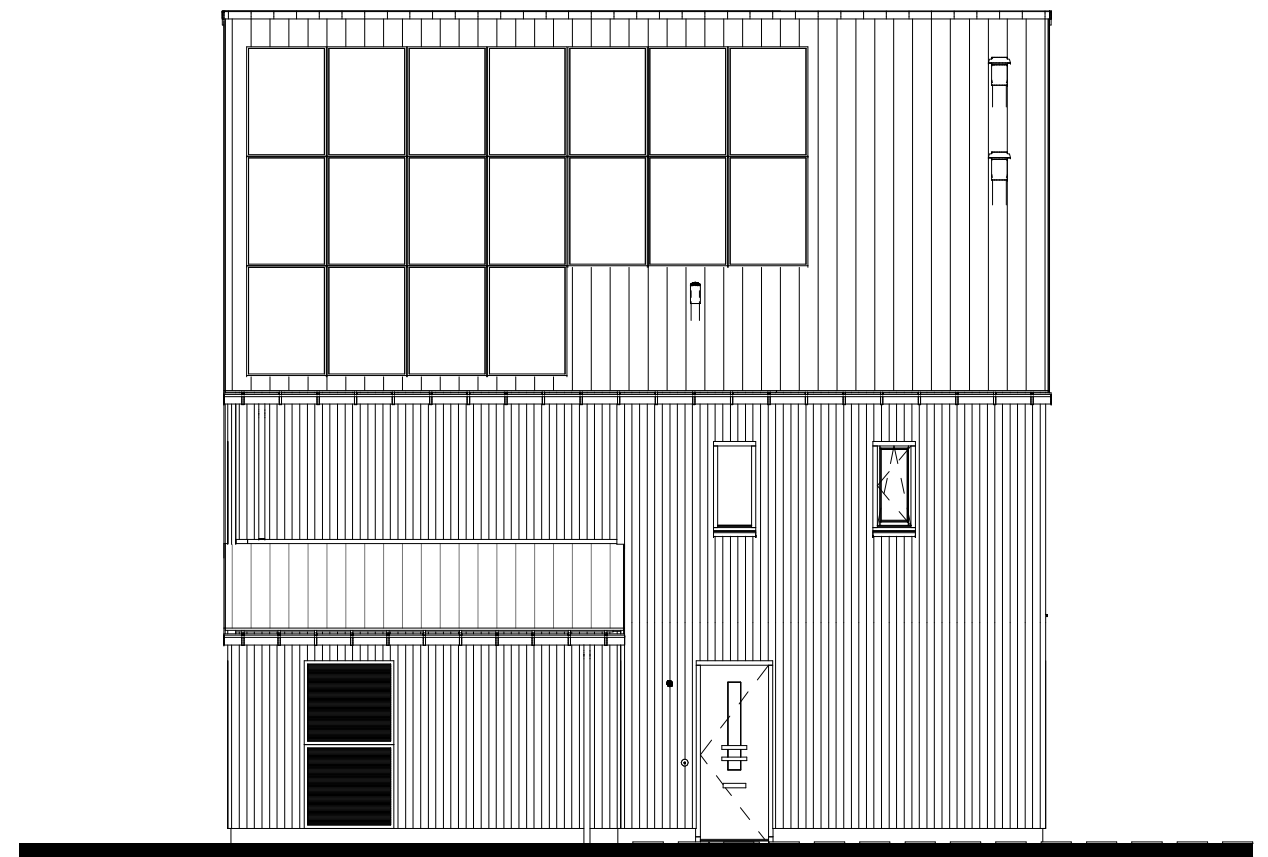
Linkerzijgevel
