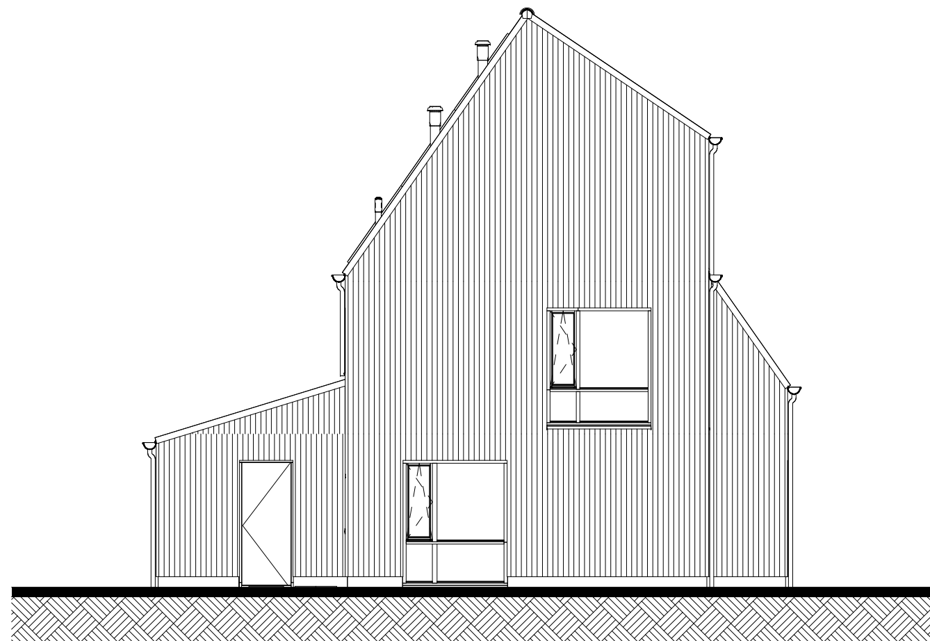
Voorgevel
