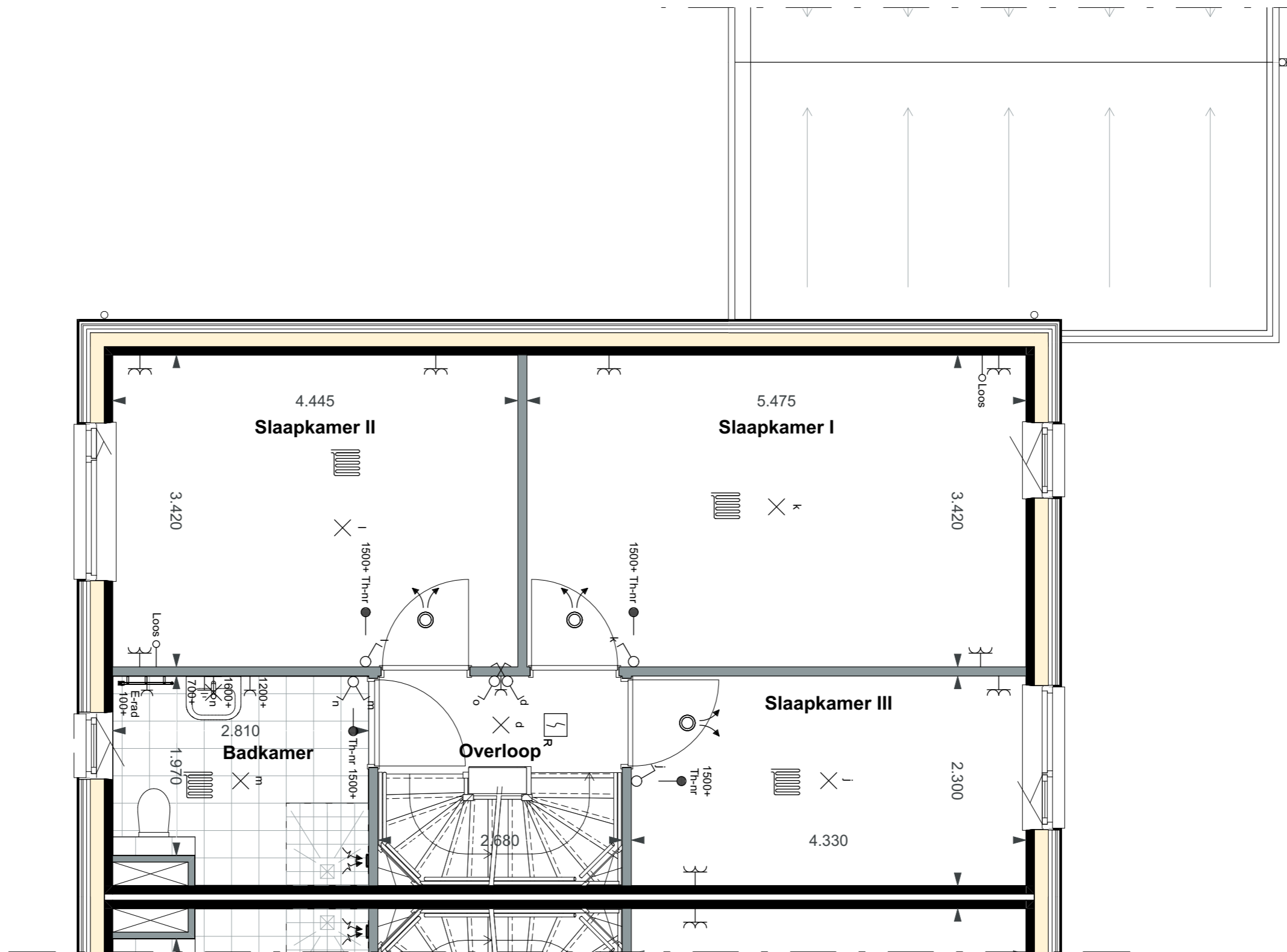
Het Bolwerk | Basistekeningen bouwnummer 52 PLG - Eerste verdieping
