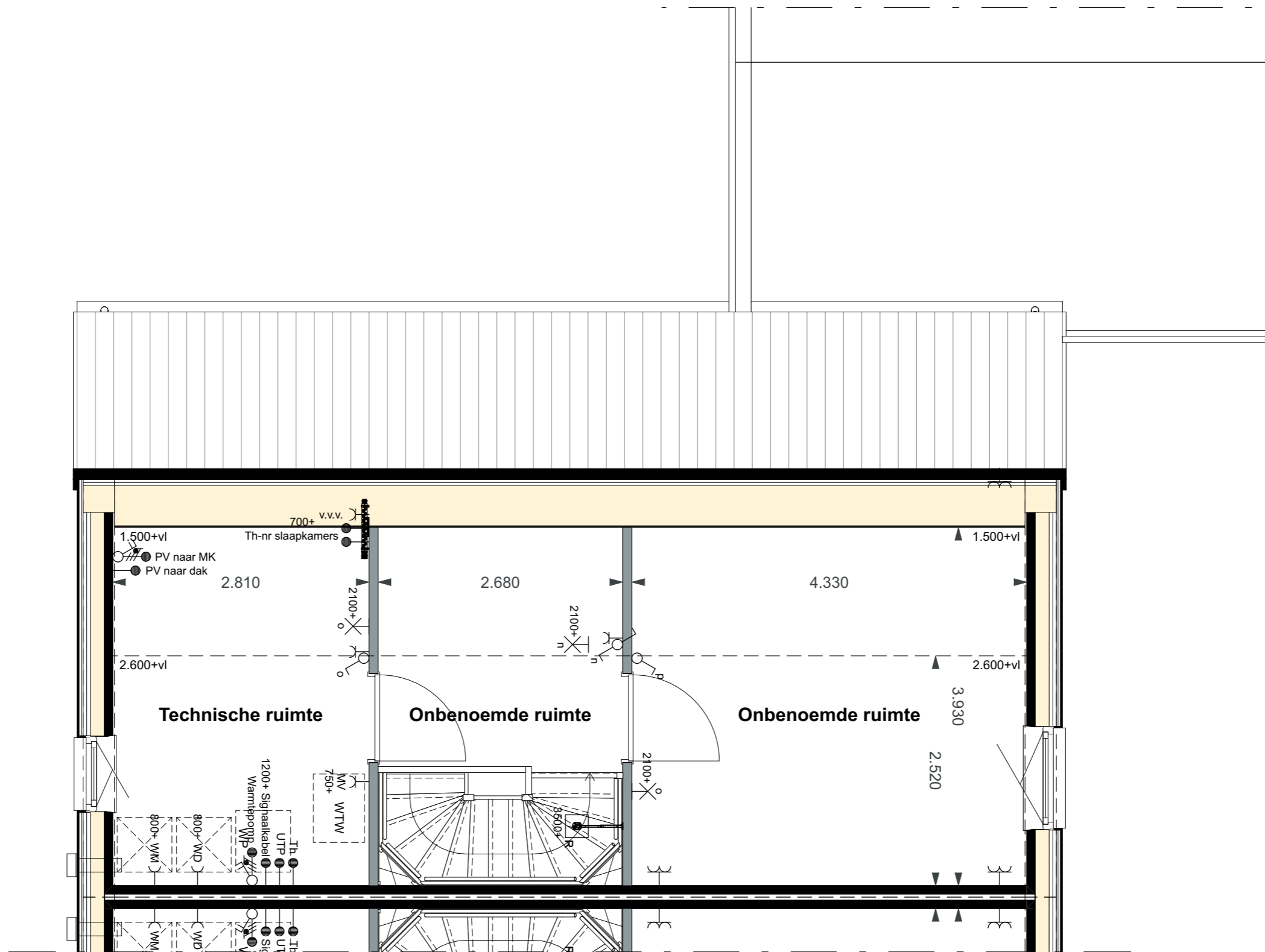
Het Bolwerk | Basistekeningen bouwnummer 52 PLG - Tweede verdieping
