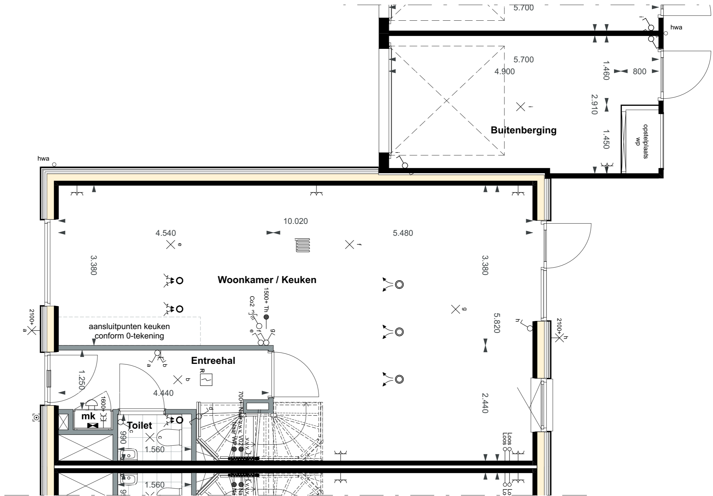
Het Bolwerk | Basistekeningen bouwnummer 52 PLG - Begane grond
