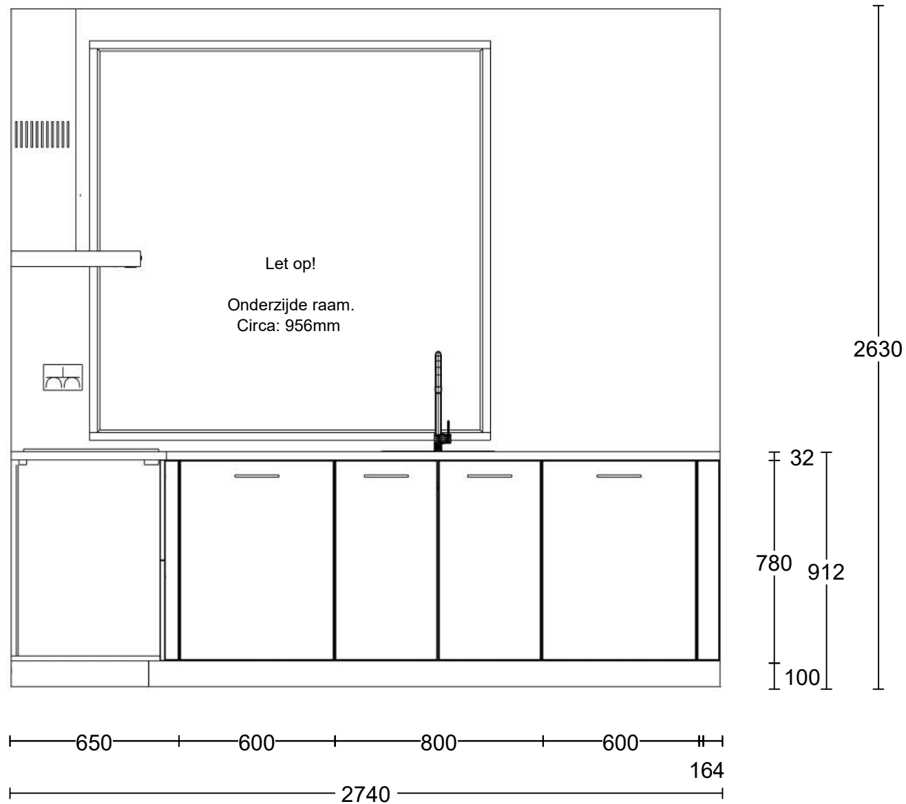
Vooraanzicht wand 2
