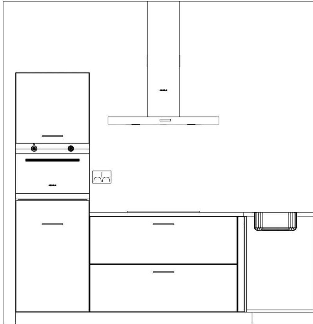
Vooraanzicht wand 1
