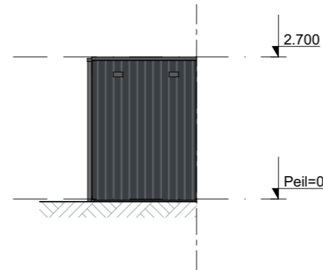
Buitenberging - Type 2 Dubbel GVL - Voorgevel
