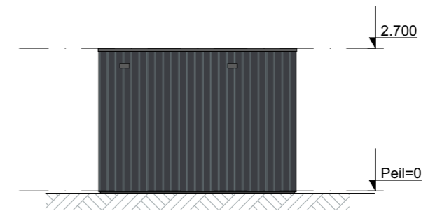
Buitenberging - Type 3 Enkel GVL - Linkergevel
