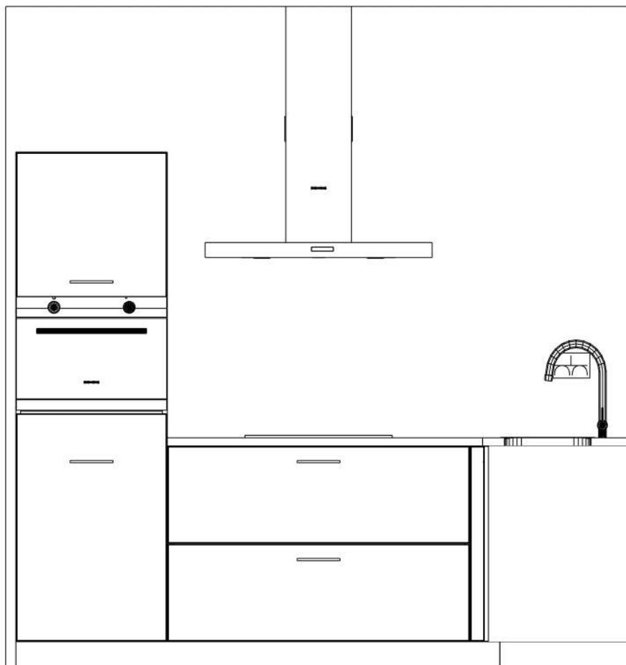
Voorraanzicht wand 1
