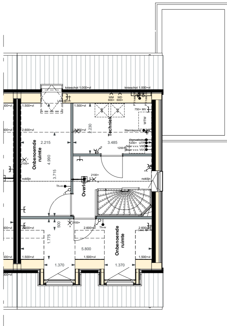
2.C.0.50 | Indelingsvariant tweede verdieping
