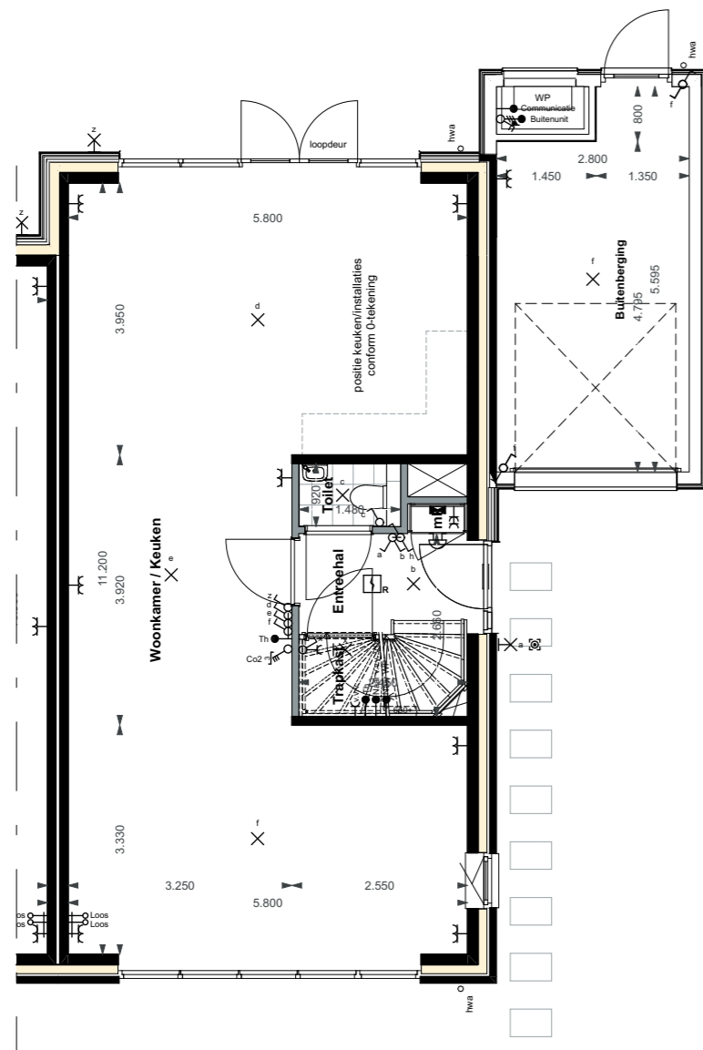
1.A.0.32 | Uitbouw achtergevel 120 cm 2.C.0.16 | Trapkast
