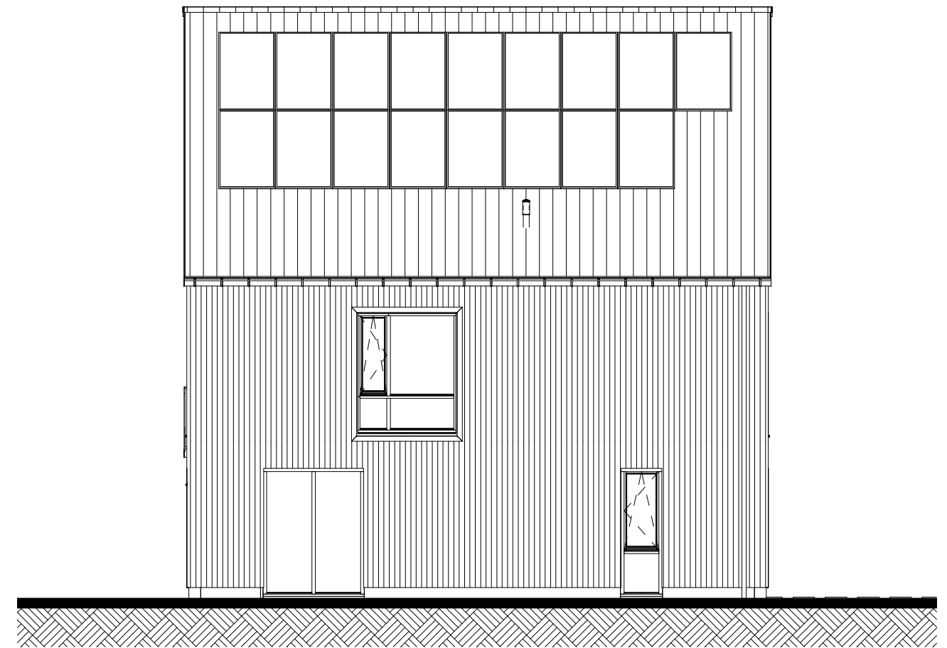
Linkergevel
