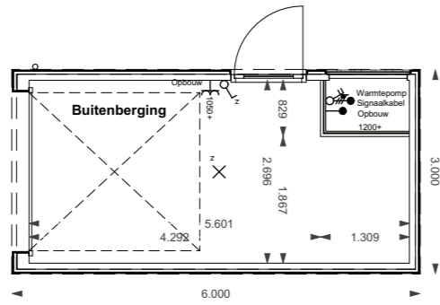
Buitenberging - type XL PLG - Begane grond
