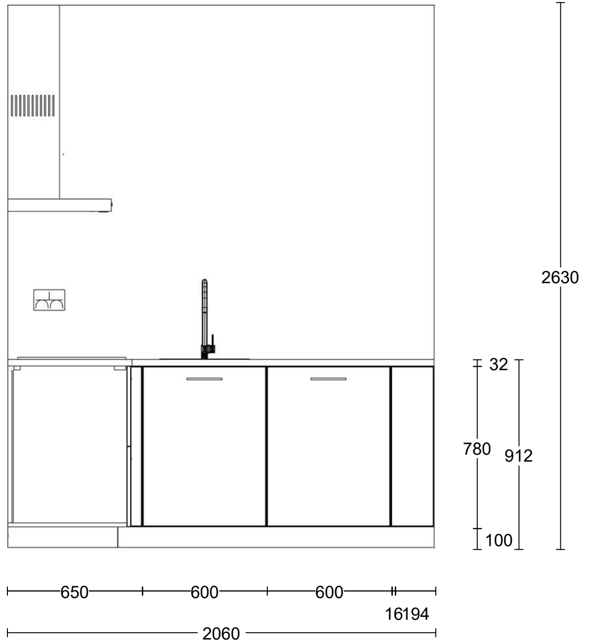
Vooraanzicht wand 2
