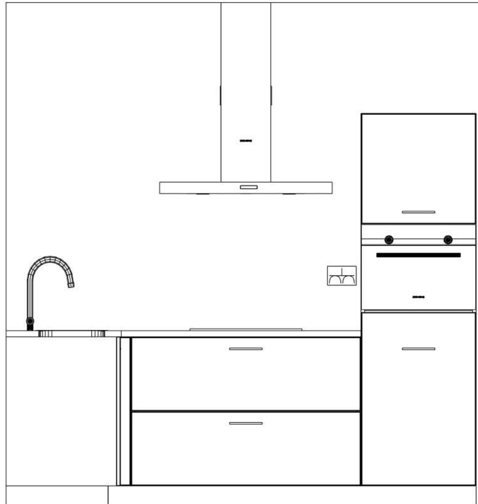
Vooraanzicht wand 2
