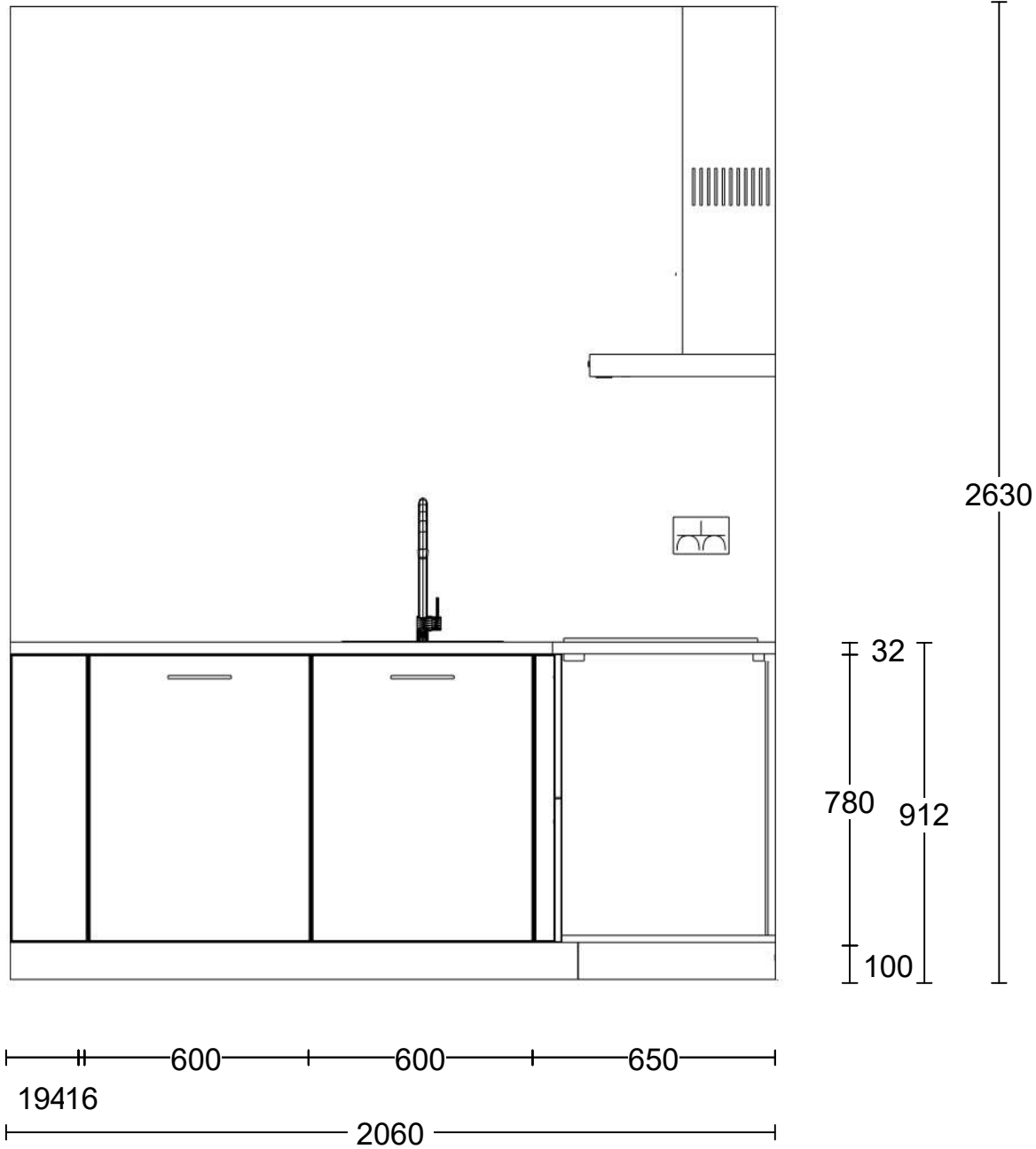
Vooraanzicht wand 1
